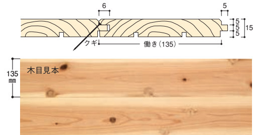
断面図 ●15mm厚 135mm巾 単位:mm
