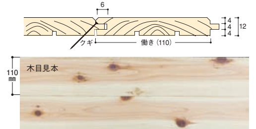
断面図 ●12mm厚 110mm巾 単位:mm
